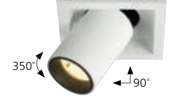
41-09-0072 3인치 엘보 사각 매입등 Size W90XH120 /타공 ø75x75 Lamp LED COB 12W / 3000K, 4000K Color 화이트
