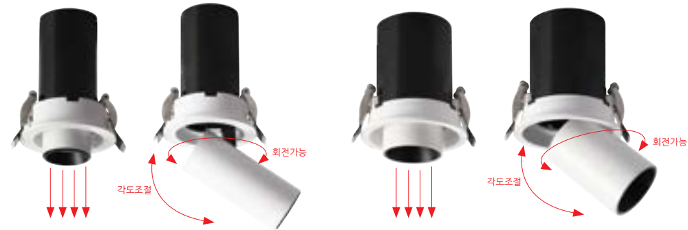
44-01-0072 LED 폴링 2인치 COB6W Size W65XD65XH95 / 타공 ø55 Lamp LED COB 6W / 3000K, 4000K Color 화이트
