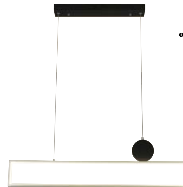
175-02-0284 포커스 1등 P/D Size W800XD20XH215 Lamp LED 40W / 4000K Color 골드+블랙
