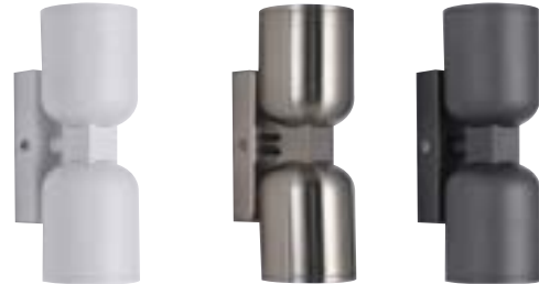
236-03-0108 (화이트, 다크그레이), 04-0116 (니켈샤틴) 프린 2등 B/R (실내외겸용 IP65) Size W63XD83XH175 Lamp LED COB 6W / 3000K Color 화이트, 다크그레이, 니켈샤틴 *LED 전용 스위치 디밍가능
