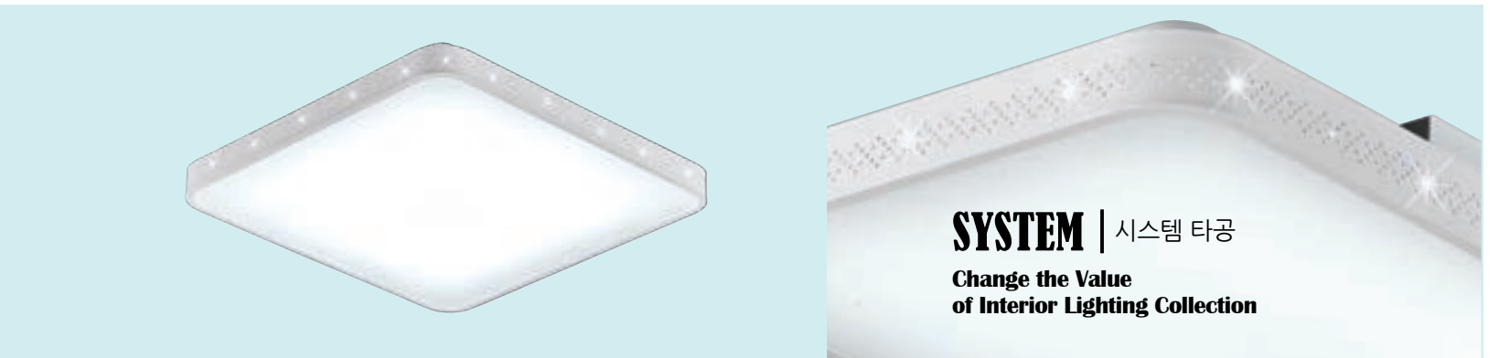
77-04-0048 시스템 타공 방등 Size W500XD500XH75 Lamp LED 50W / 6500K Color 화이트
