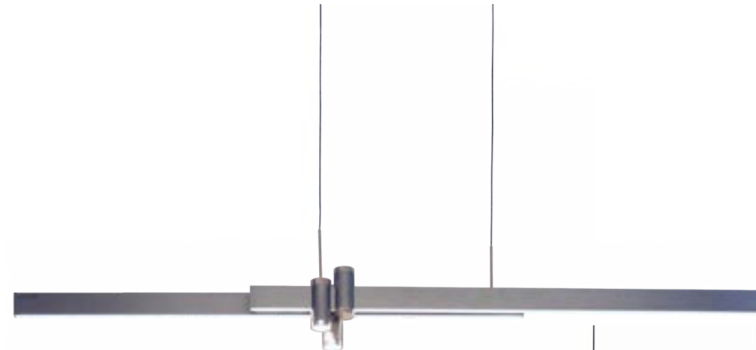
129-01-0396 제타 P/D Size W1280XD 60XH120 Lamp LED 40W / 4000K Color 실버그레이
