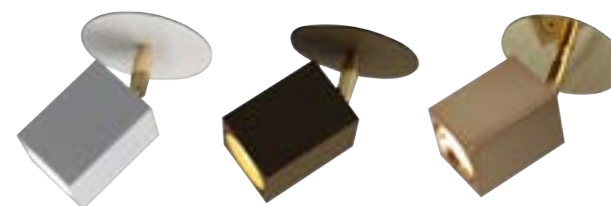
189-10-0108 (골드) 189-11-0090 (코랄, 민트, 모카) 189-12-0084 (화이트, 블랙) 앵거 매입직부 V타입 85 / 타공 ø75 Size W60XD60XH150 Lamp LED GU10X1
