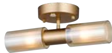
196-13-0104 (센서), 14-0096 (직부) 나르샤 2등 센서/직부 Size W340XD130XH130 Lamp LED G9X2 Color 브론즈+유리
