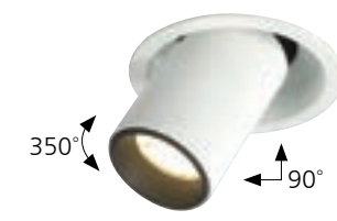
41-08-0072 3인치 엘보 원형 매입등 Size W85XH120 /타공 ø75 Lamp LED COB 12W / 3000K, 4000K Color 화이트
