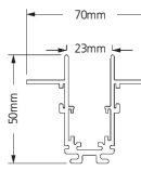
50-01 매입형 레일 Size 1M, 1.5M, 2M Color 흑색
